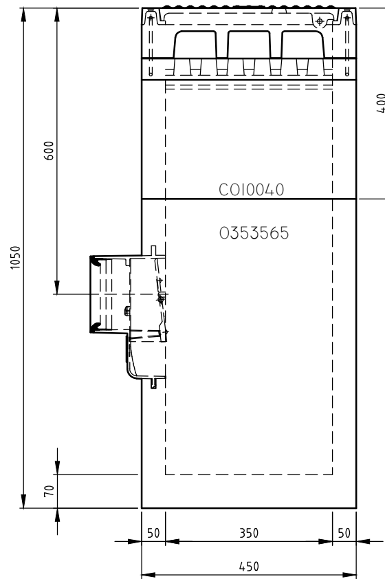
VOORAANZICHT
