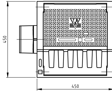
BOVENAANZICHT
