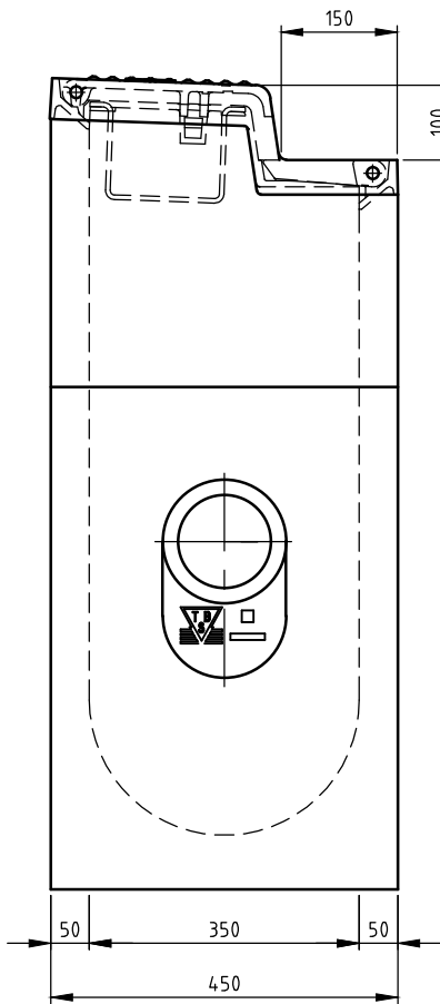
ZIJ-AANZICHT
