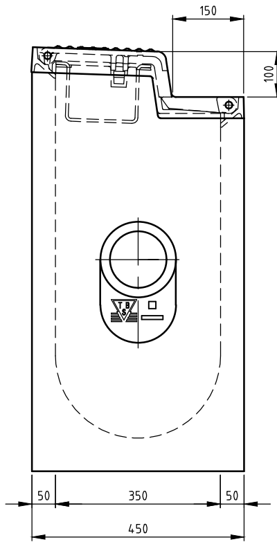
ZIJ-AANZICHT
