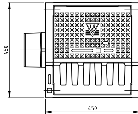
BOVENAANZICHT
