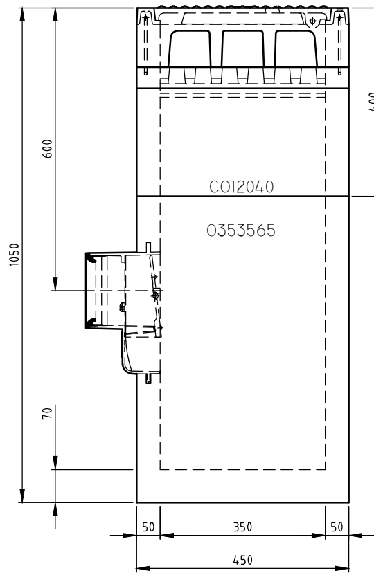
VOORAANZICHT
