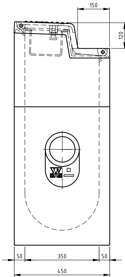
ZIJ-AANZICHT
