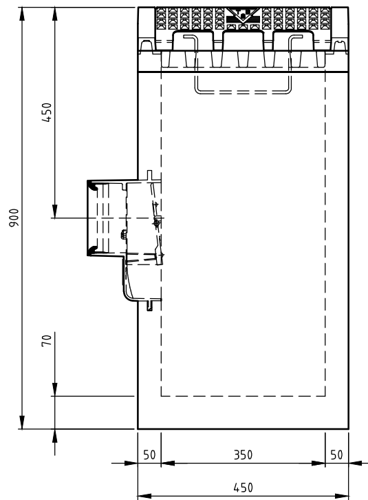
VOORAANZICHT
