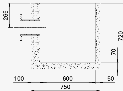
DOORSNEDE A-A
