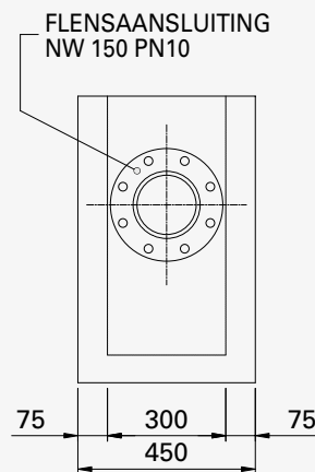
VOORAANZICHT
