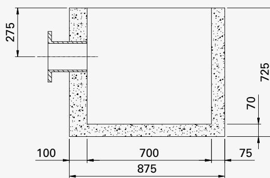
DOORSNEDE A-A
