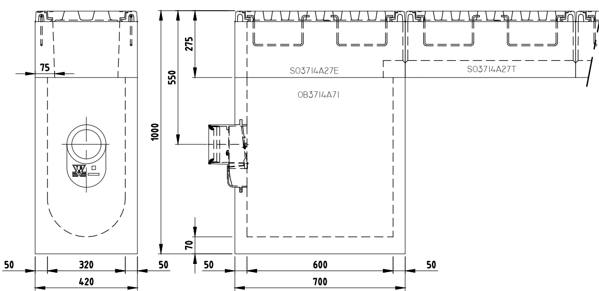
ZIJ-AANZICHT
