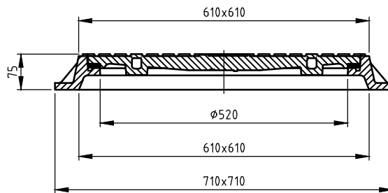
DOORSNEDE A-A
