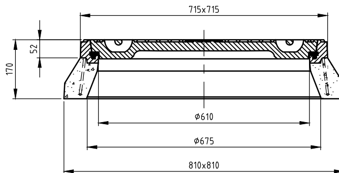
DOORSNEDE A-A
