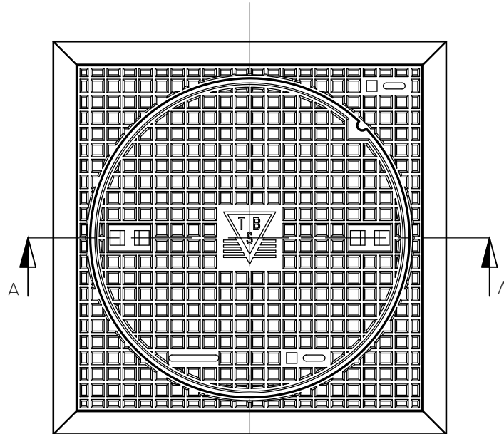
BOVENAANZICHT
