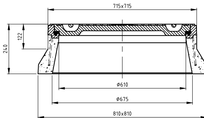
DOORSNEDE A-A
