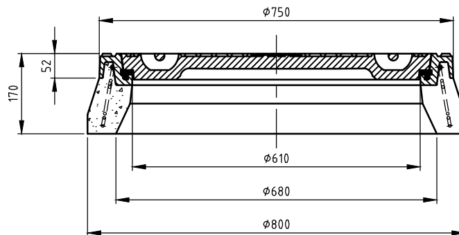
DOORSNEE A-A
