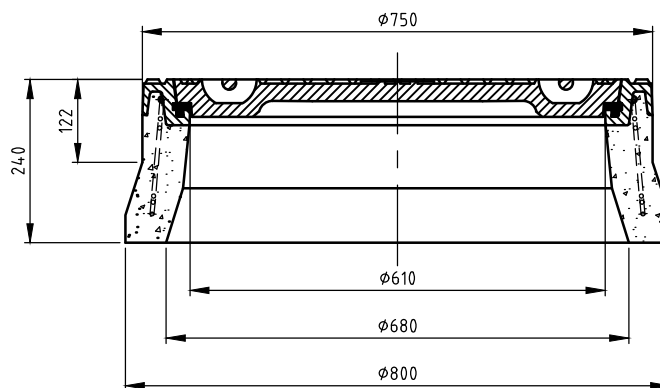
DOORSNEDE A-A
