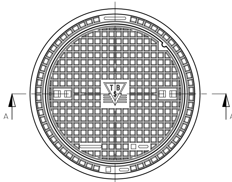
BOVENAANZICHT
