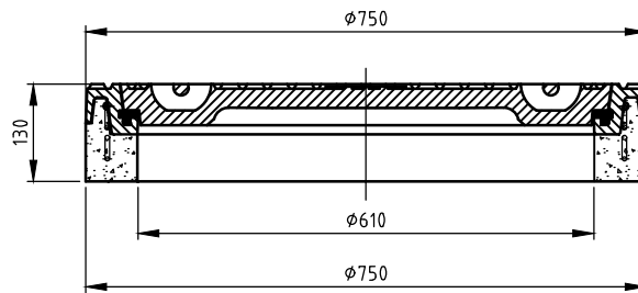
DOORSNEDE A-A
