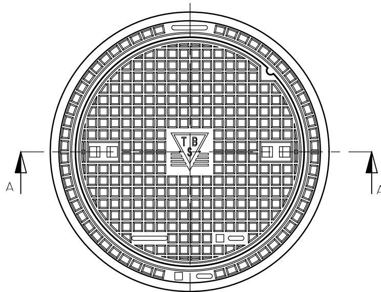
BOVENAANZICHT
