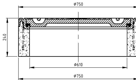
DOORSNEDE A-A
