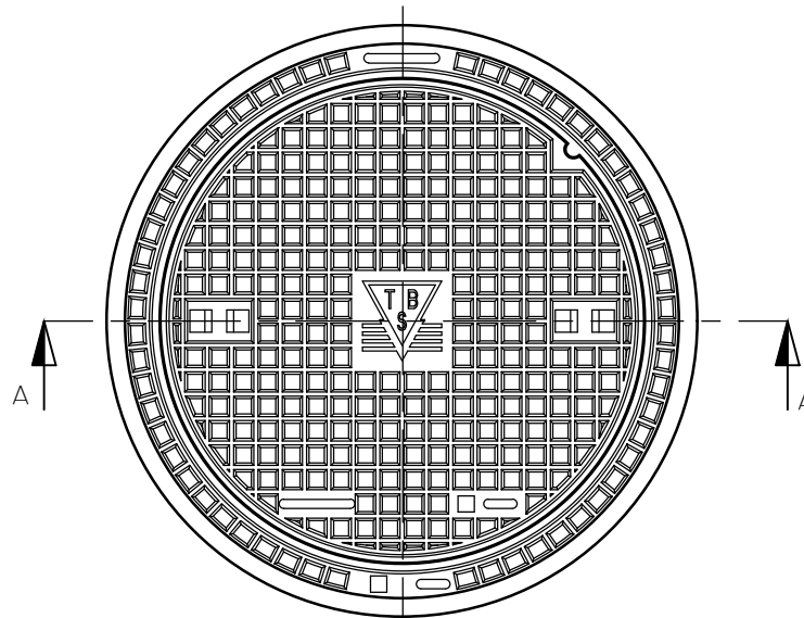
BOVENAANZICHT
