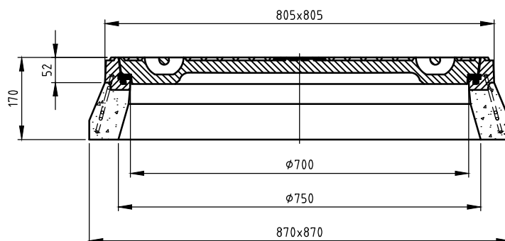
DOORSNEDE A-A
