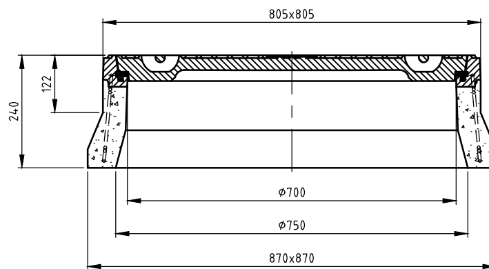
DOORSNEDE A-A
