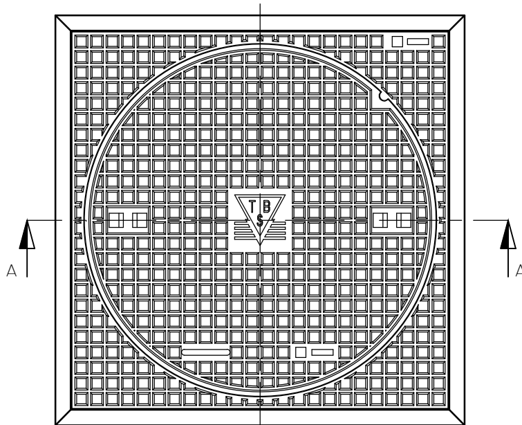
BOVENAANZICHT
