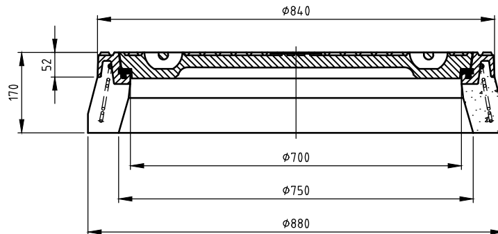
DOORSNEDE A-A
