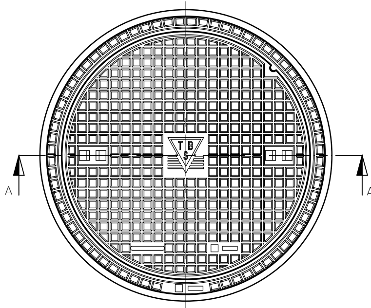
BOVENAANZICHT
