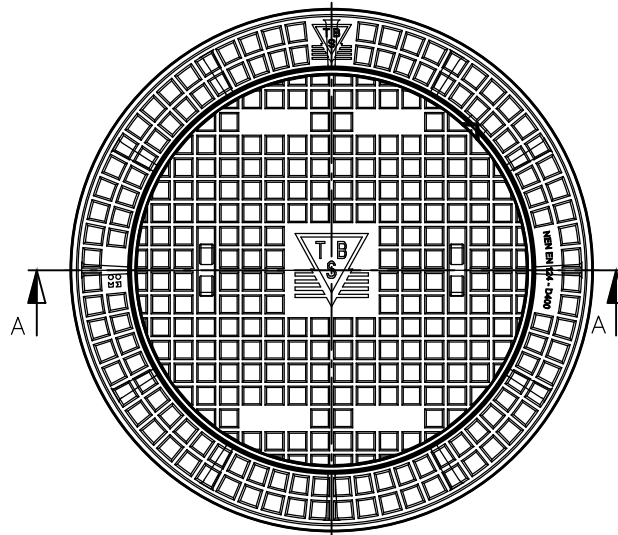
BOVENAANZICHT
