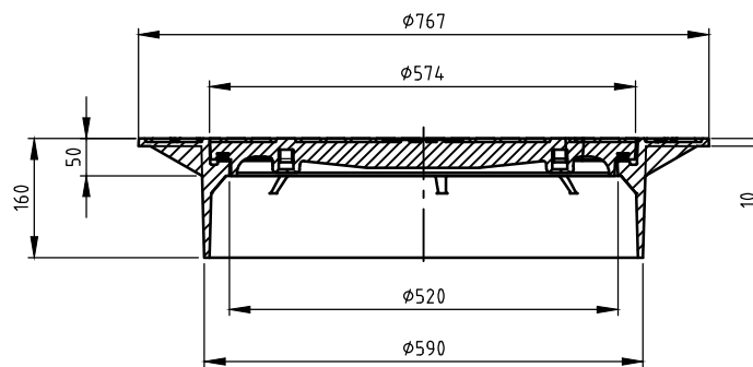
DOORSNEDE A-A
