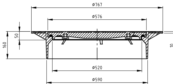
DOORSNEDE A-A
