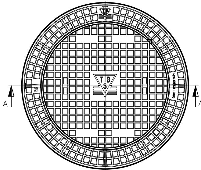
BOVENAANZICHT
