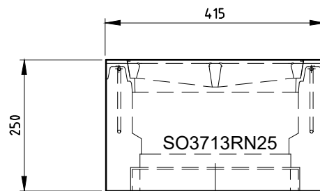
BOVENAANZICHT
