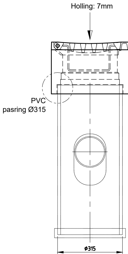
zij-aanzicht
