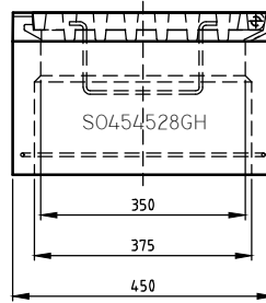
BOVENAANZICHT
