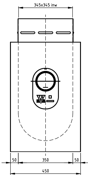
ZIJ-AANZICHT
