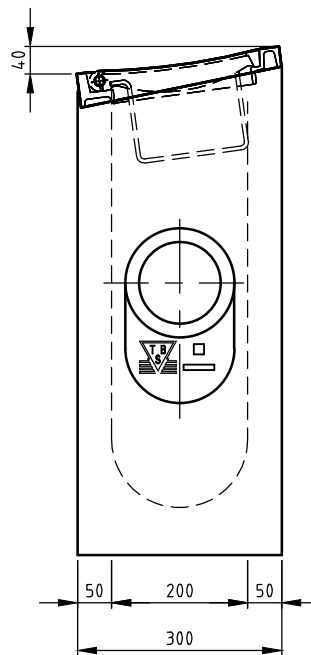
ZIJ-AANZICHT
