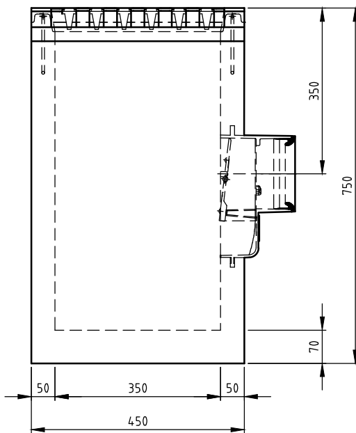
ACHTERAANZICHT
