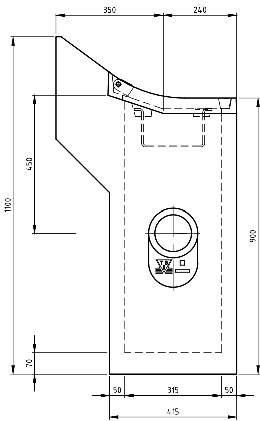
ZIJ-AANZICHT
