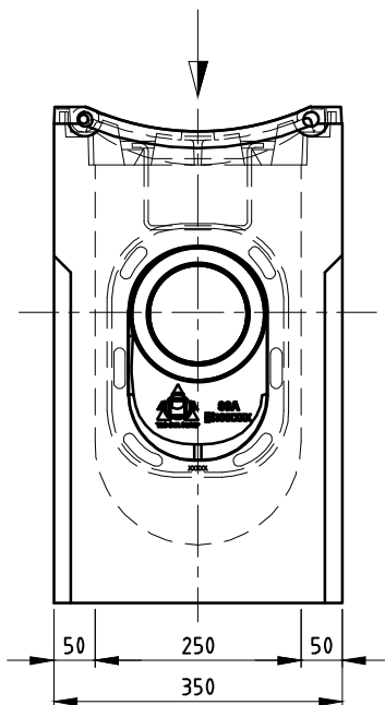
ZIJAANZICHT
