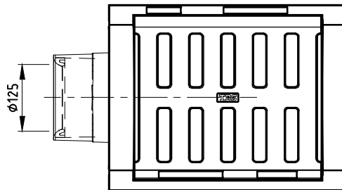
BOVENAANZICHT
