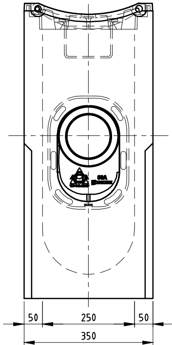
ZIJAANZICHT
