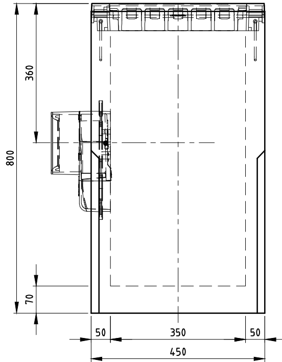
VOORAANZICHT
