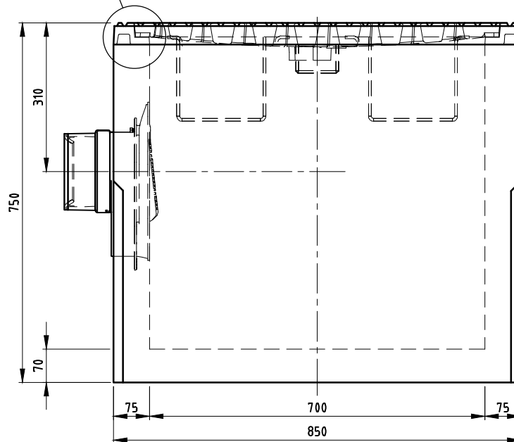
VOORAANZICHT
