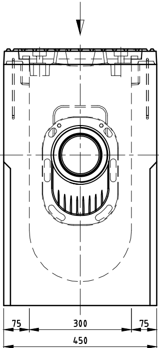
ZIJAAANZICHT
