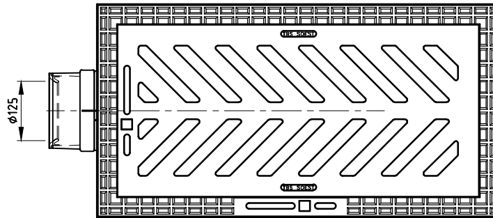
BOVENAANZICHT
