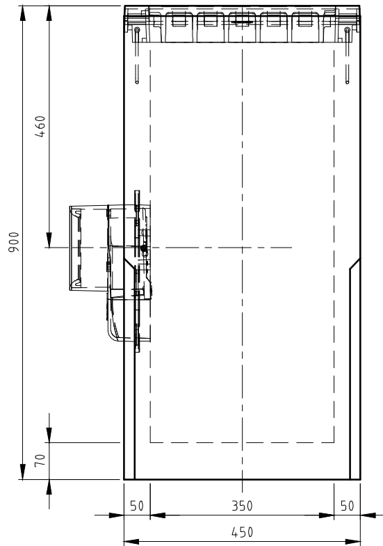
VOORAANZICHT
