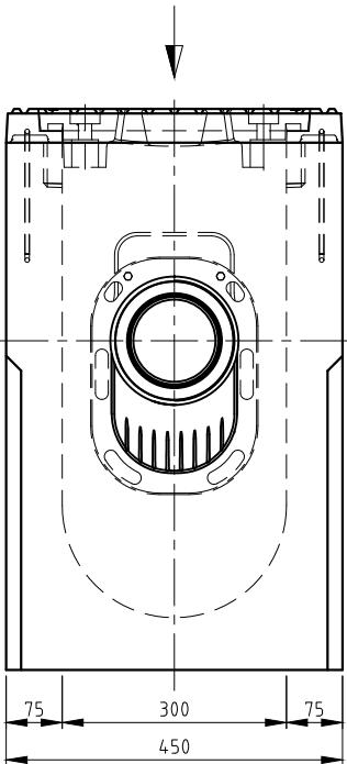
ZIJAAANZICHT
