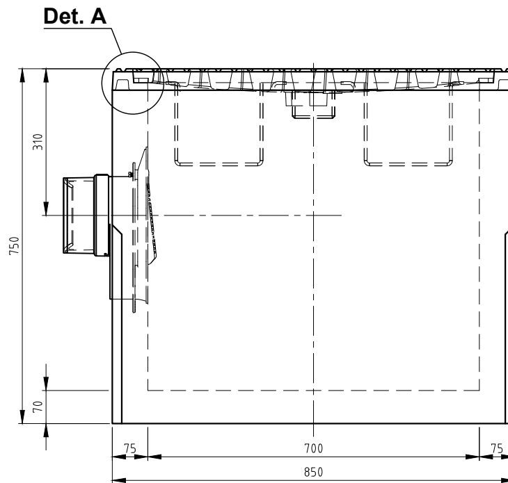
VOORAANZICHT
