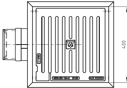
BOVENAANZICHT
