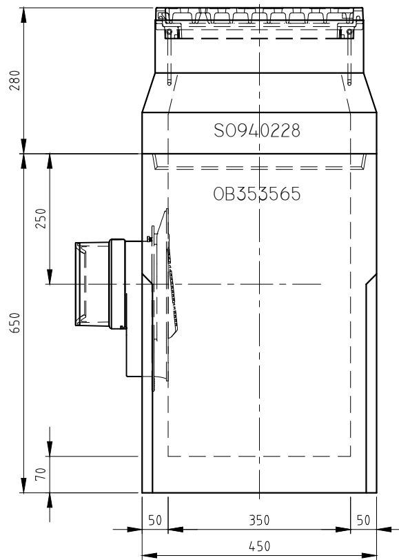
VOORAANZICHT
