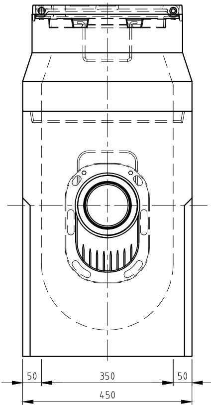
ZIJAAANZICHT
