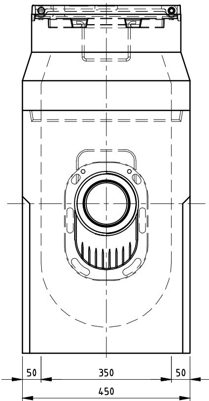
ZIJAANZICHT
