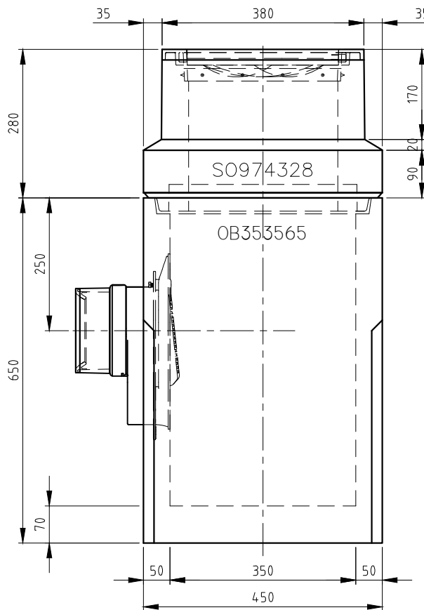
VOORAANZICHT
