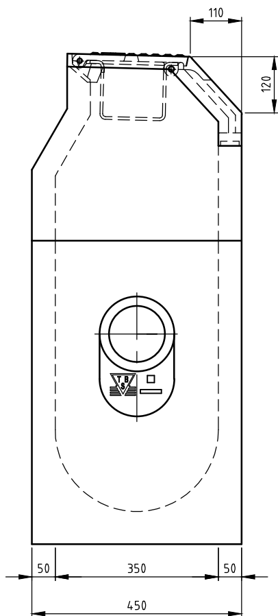
ZIJ-AANZICHT
