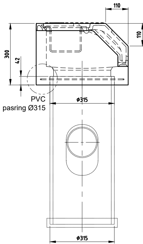
zij-aanzicht
