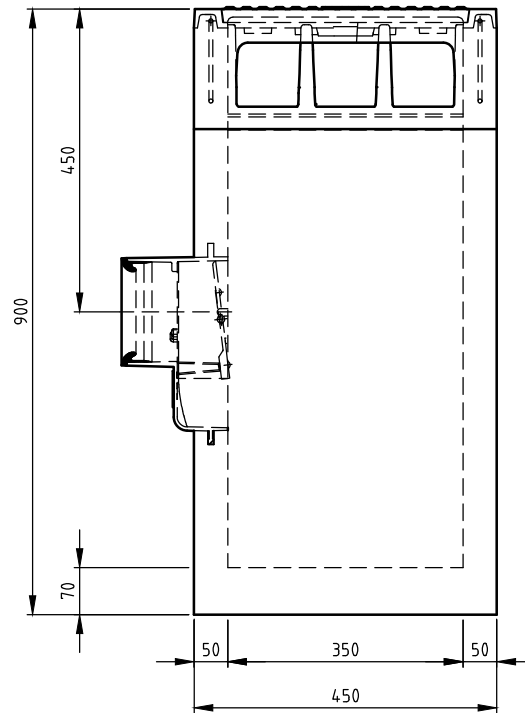
VOORAANZICHT
