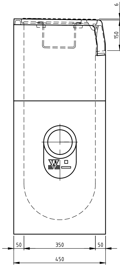
ZIJ-AANZICHT
