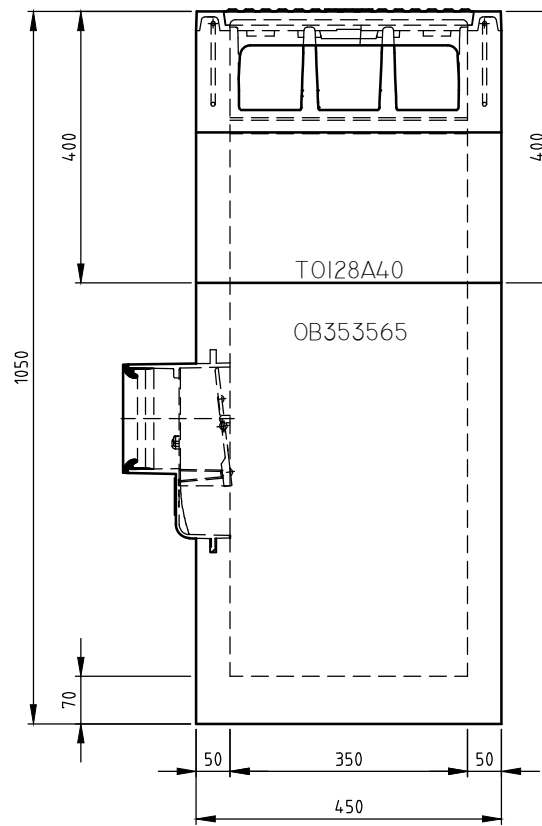
VOORAANZICHT
