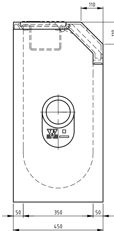
ZIJ-AANZICHT
