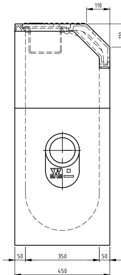
ZIJ-AANZICHT
