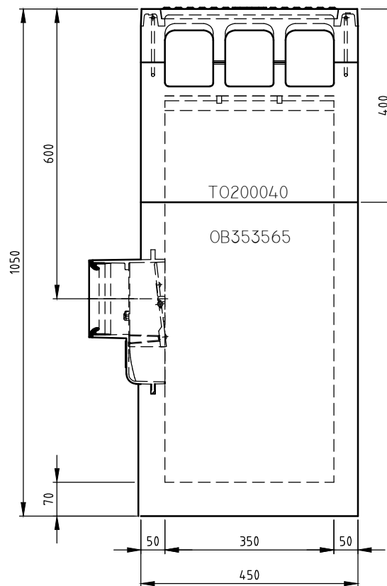
VOORAANZICHT
