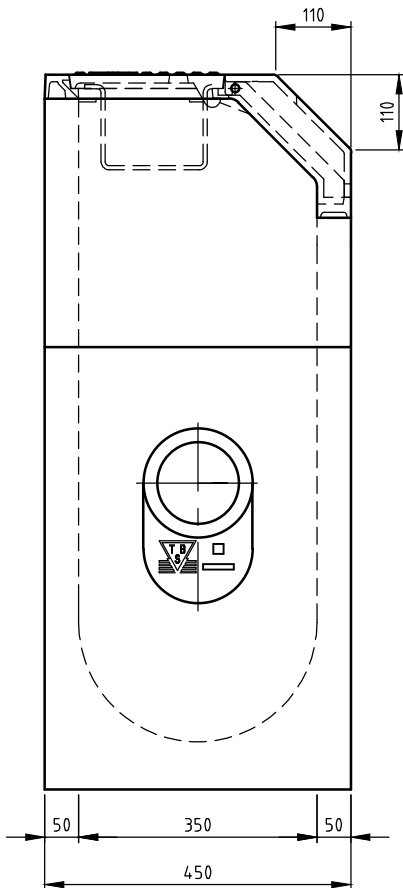
ZIJ-AANZICHT
