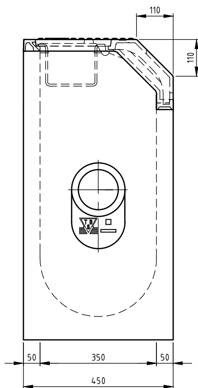
ZIJ-AANZICHT
