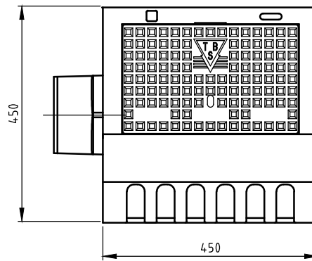
BOVENAANZICHT
