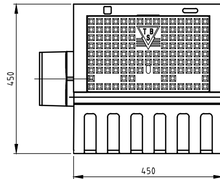
BOVENAANZICHT
