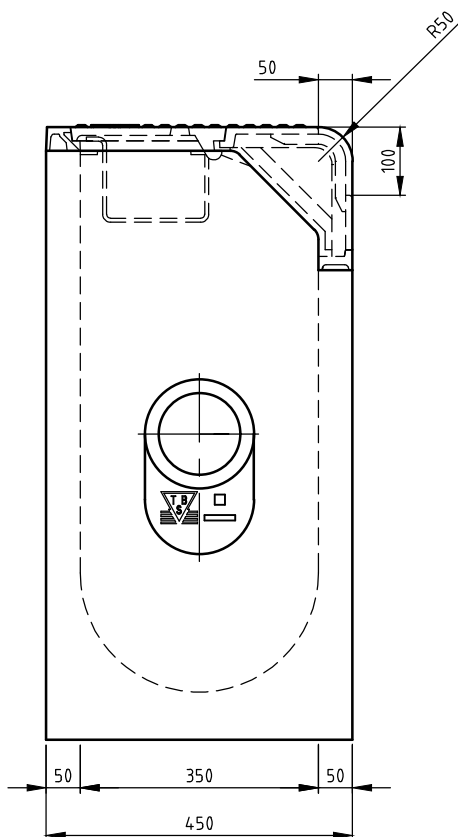
ZIJ-AANZICHT
