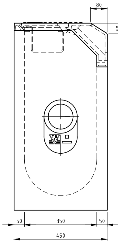
ZIJ-AANZICHT
