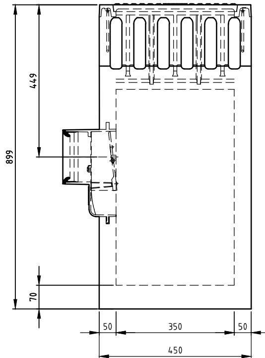
VOORAANZICHT
