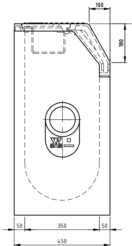
ZIJ-AANZICHT
