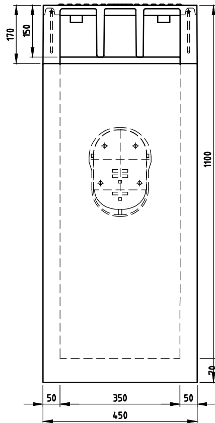
VOORAANZICHT
