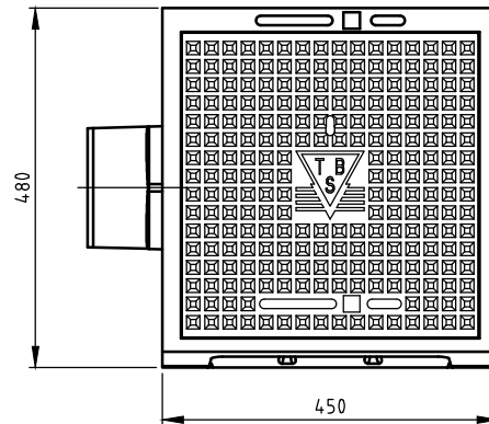
BOVENAANZICHT
