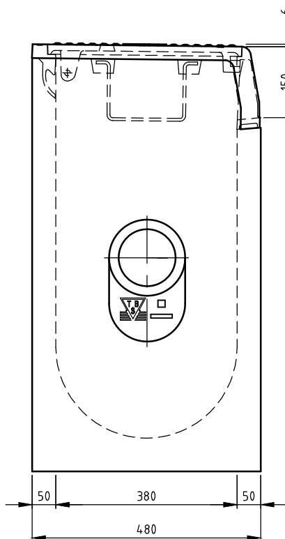
ZIJ-AANZICHT
