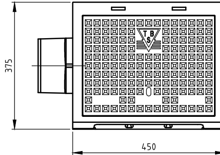
BOVENAANZICHT
