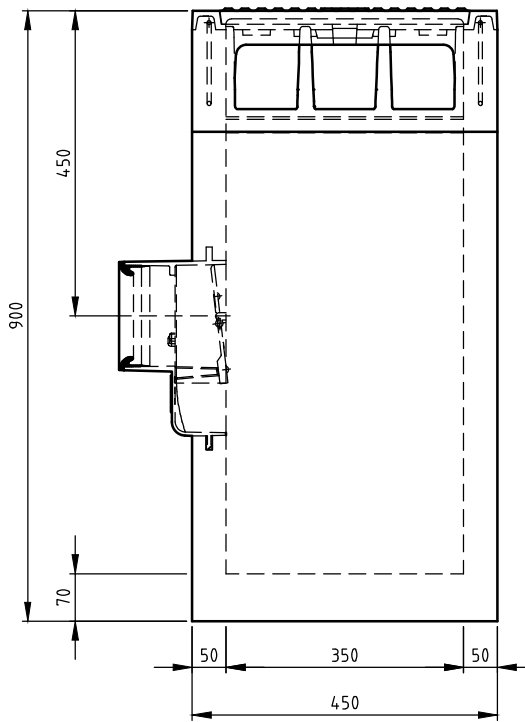
VOORAANZICHT
