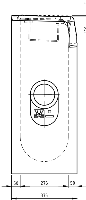
ZIJ-AANZICHT
