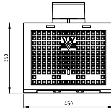
BOVENAANZICHT
