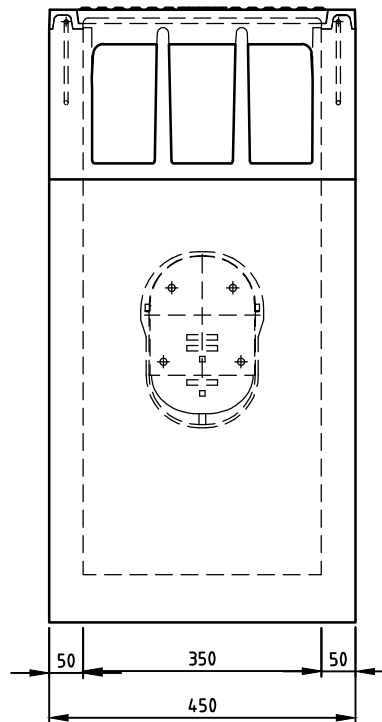
VOORAANZICHT
