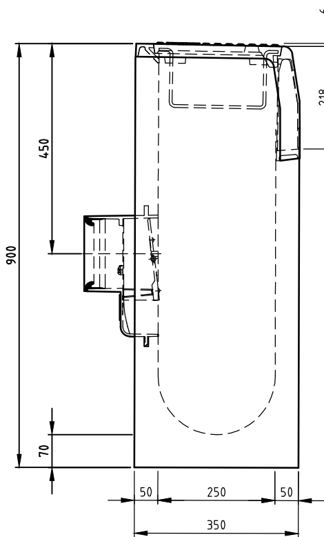
ZIJ-AANZICHT
