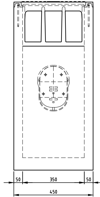
VOORAANZICHT
