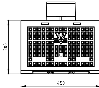
BOVENAANZICHT
