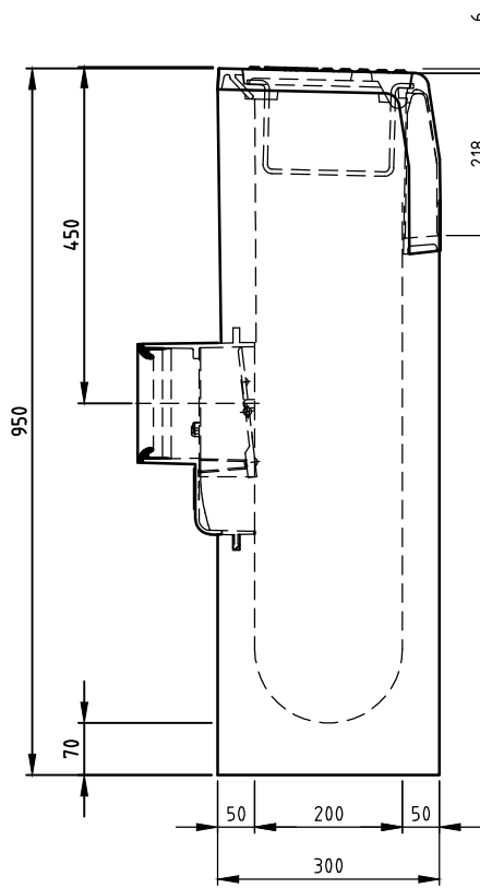
ZIJ-AANZICHT
