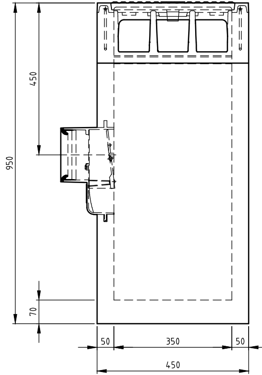
VOORAANZICHT
