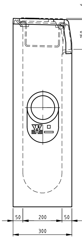
ZIJ-AANZICHT
